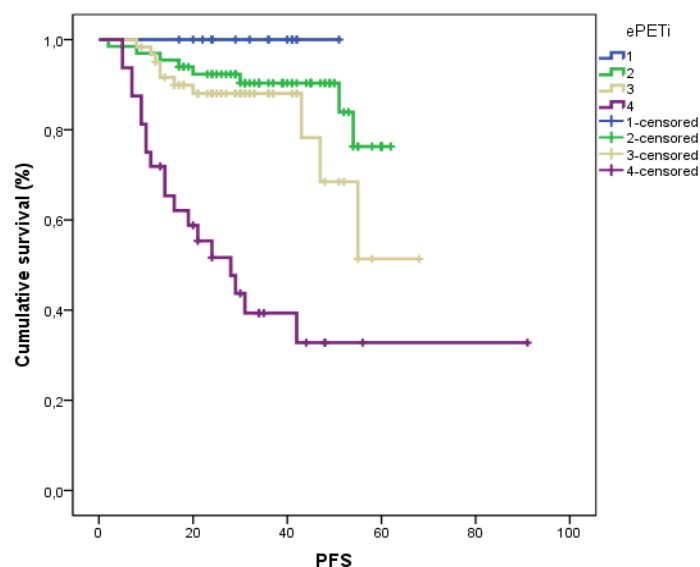
Función de supervivencia libre de enfermedad acumulada respecto del estado metabólico en pacientes con cáncer de pecho localmente avanzado.
