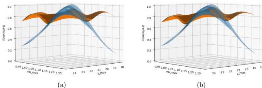
Análisis de eficiencias del diseño D-óptimo (azul) y los diseños aumentados en 2 puntos (a) y en 4 puntos (b).
